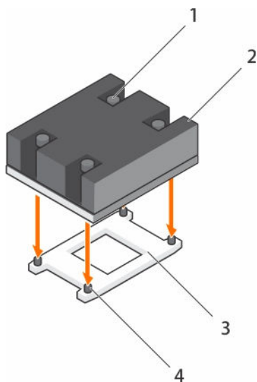
図 36. ヒートシンクの取り付け
