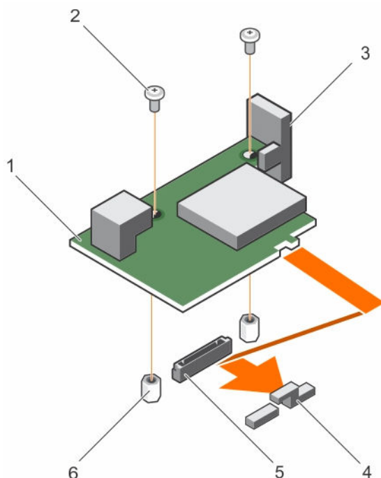
図 25. IDSDM カードの取り付け
