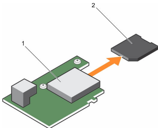
図 21. SD カードの取り付け
