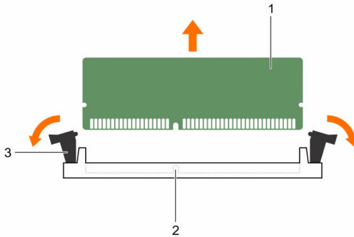
図 15. メモリモジュールの取り外し
