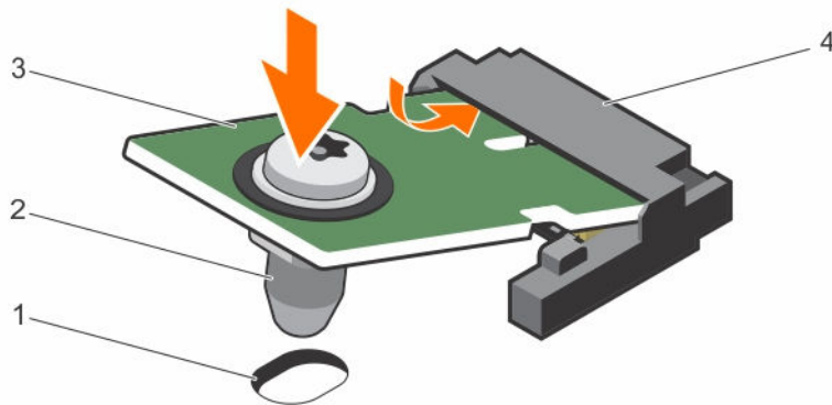
図 71. TPM の取り付け
