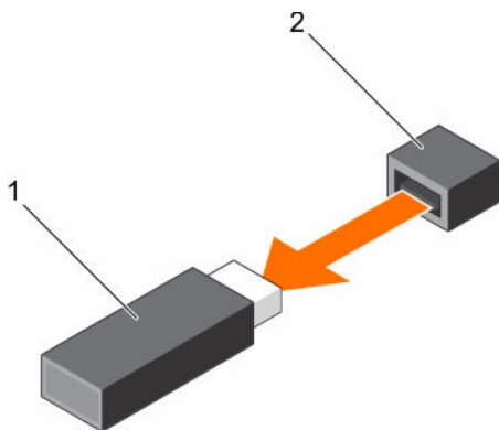
図 22. 内蔵 USB メモリキーの取り外し
