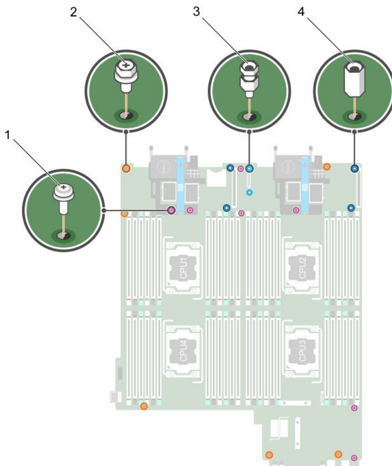
図 68. システム基板上的異なる種類のネジ
