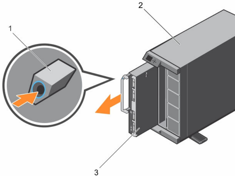
図 6. サーバーモジュールの取り外し
