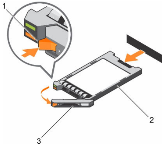
図 41. SSD の取り外し
