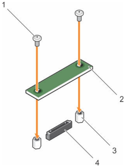
図 27. rSPI カードの取り付け
