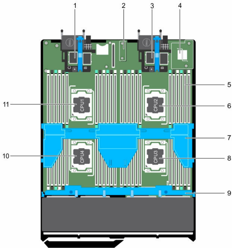
図 10. サーバーモジュールの内部
