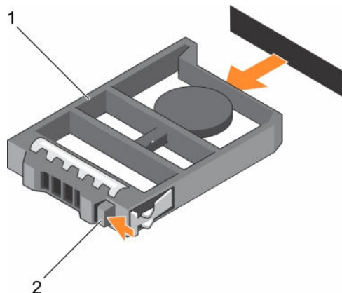
図 44. 2.5 インチのハードドライブダミーの取り外し
