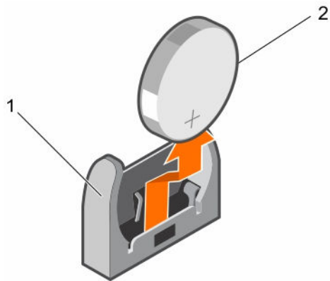
図 62. NVRAM バックアップバッテリーの取り外し
