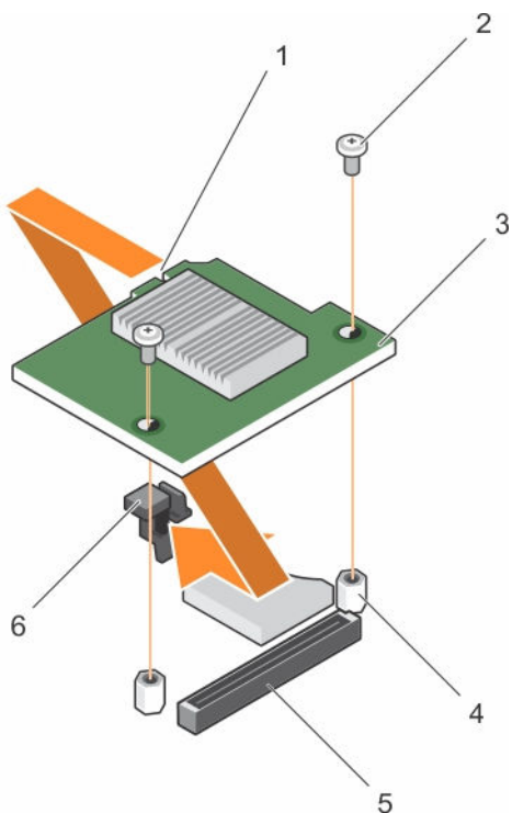
図 31. NDC の取り付け
