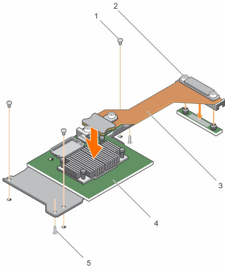
図 67. エキスパンダカードの取り付け
