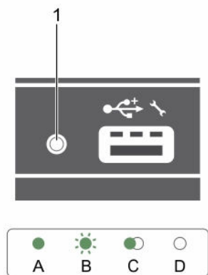
図 5. iDRAC Direct LED インジケータ
