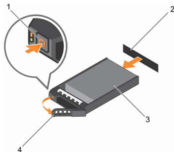
図 40. ハードドライブの取り外し
