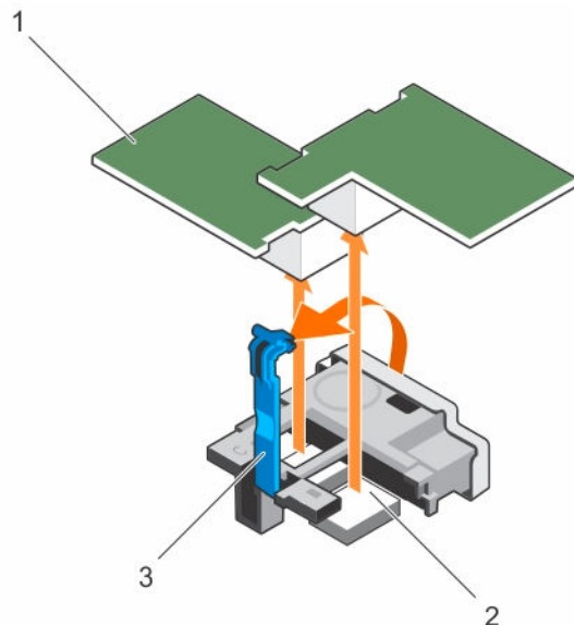
図 17. PCIe メザニンカードの取り外し
