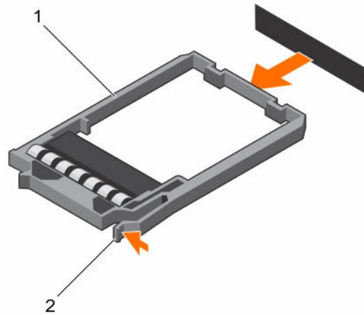
図 45.1.8 インチ SSD ダミーの取り外し
