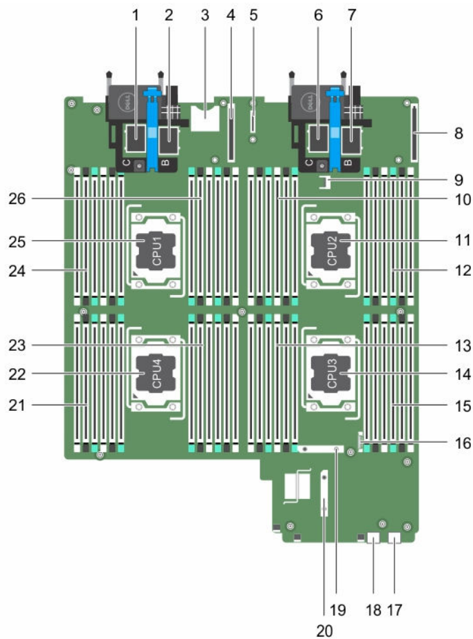
図 72. システム基板のコネクタ
