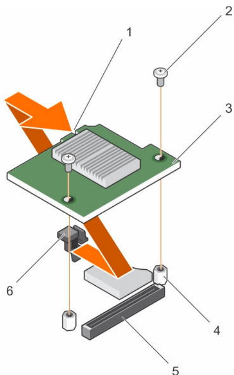
図 30. NDC の取り外し
