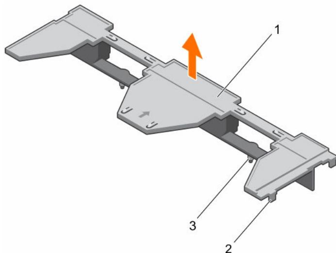
図 11. 冷却用エアフローカバーの取り外し
