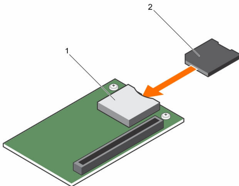
図 29. SD vFlash カードの取り付け
