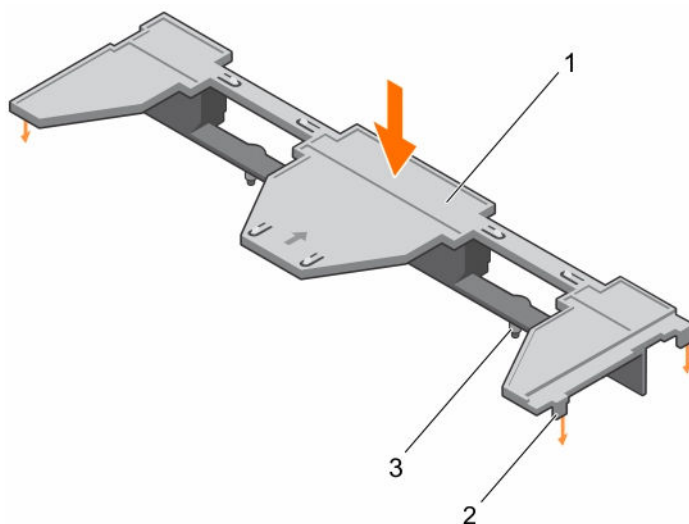
図 12. 冷却エアフローカバーの取り付け
