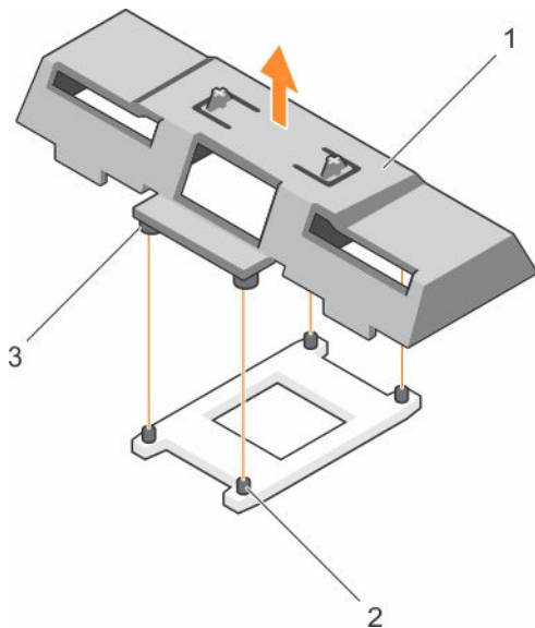
図 13. プロセッサダミー と DIMM ダミーの取り外し
