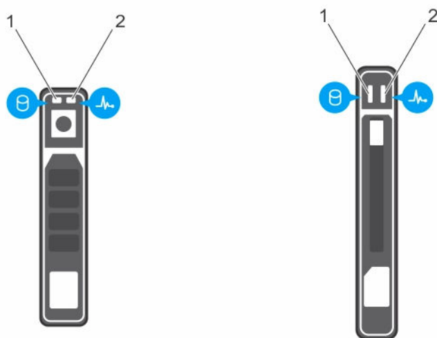
図 4. ハードドライブまたは SSD インジケータ
