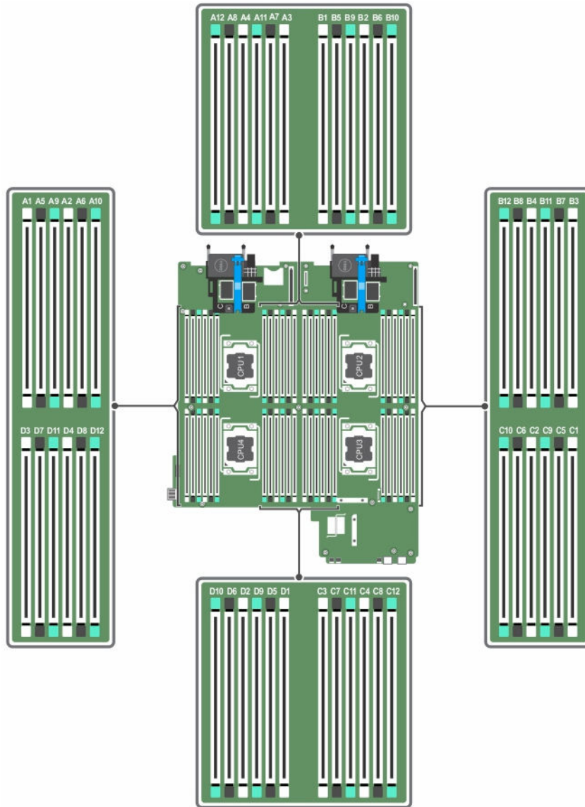
図 14. メモリソケットの位置
