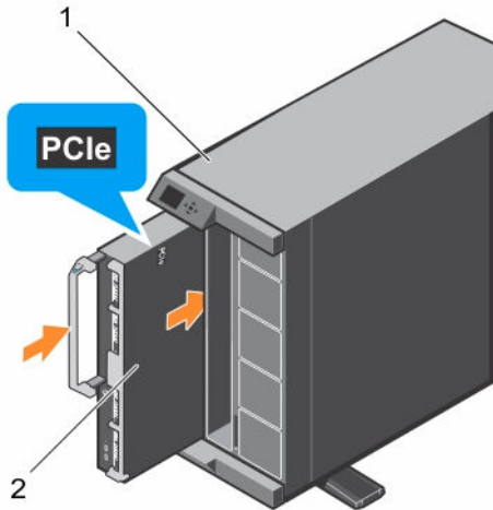
図 7. サーバーモジュールの取り付け
