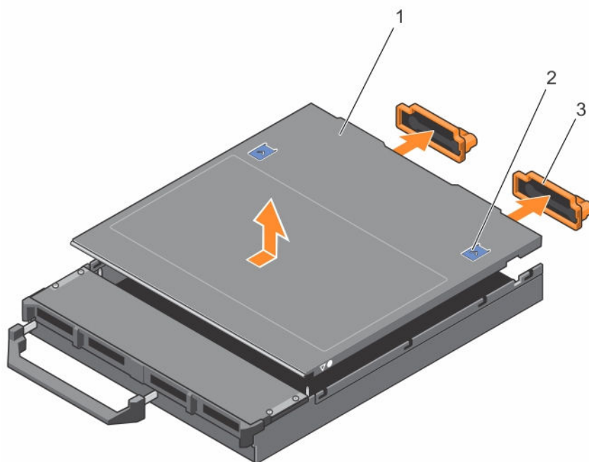
図 8. システムカバーの取り外し
