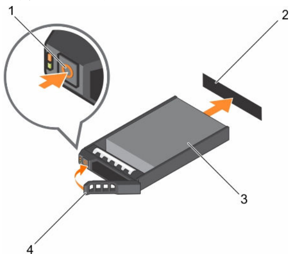
図 42. ハードドライブの取り付け
