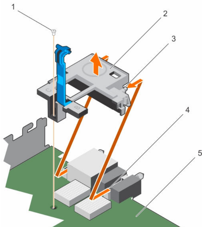
図 19. PCIe メザニカードのサポートブラケットの取り外し
