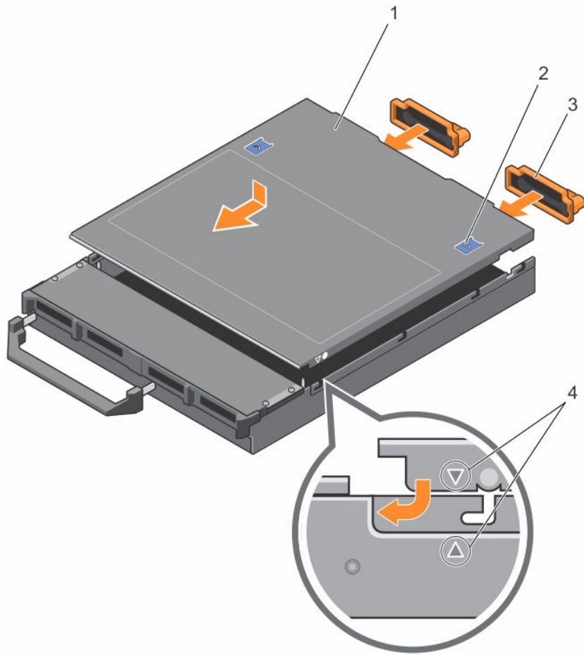
図 9. システムカバーの取り付け
