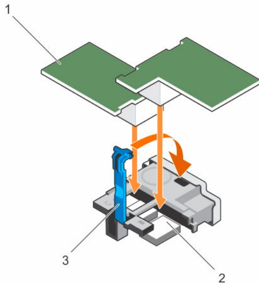
図 18. PCIe メザニンカードの取り付け
